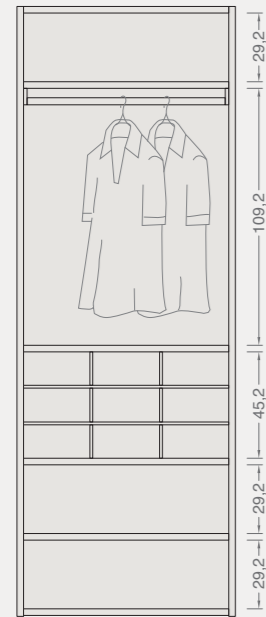
4 ripiani 1 tubo appendiabiti 1 crociera interna 4 shelves 1 coat-hanger 1 inner cruiser
